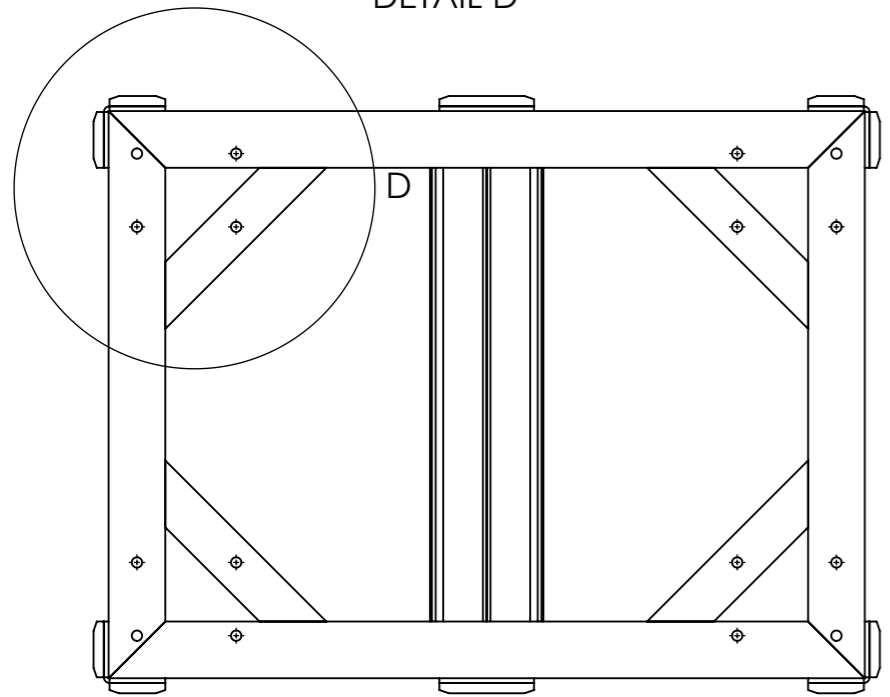
DÉTAIL D
