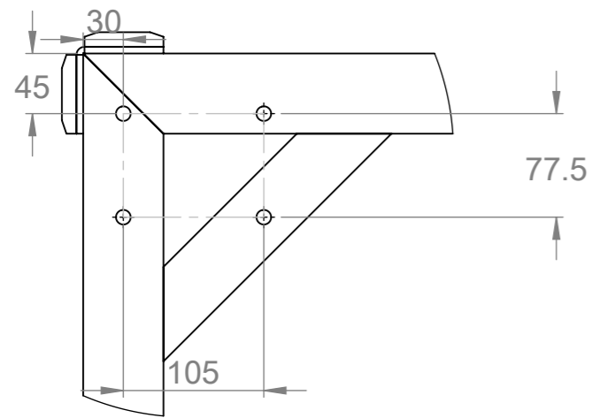
DÉTAIL C
