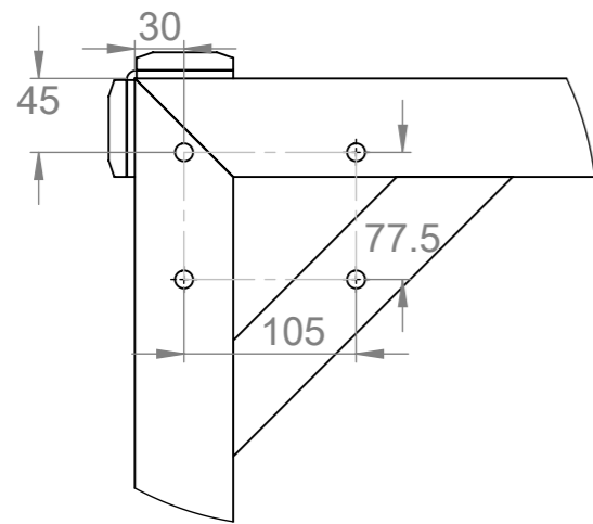
DÉTAIL D
