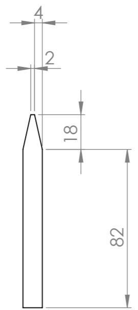
Détail de l'affutage des couteaux
