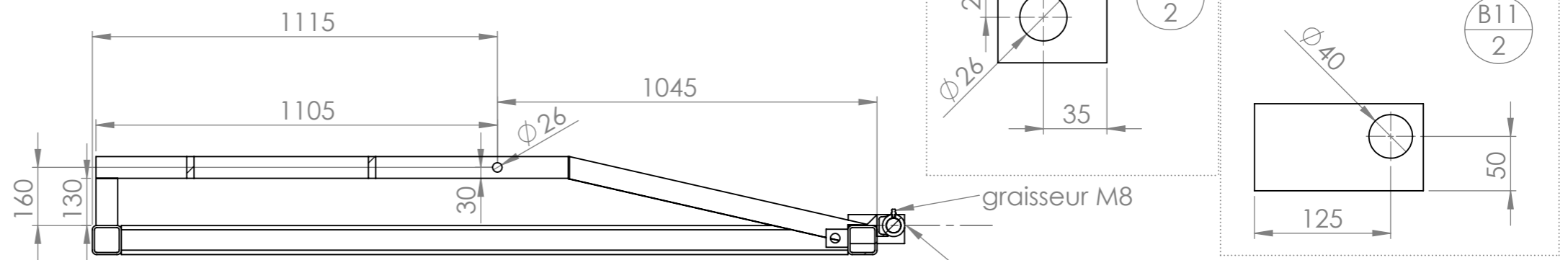
COUPE D-D ECHELLE 1 : 15
