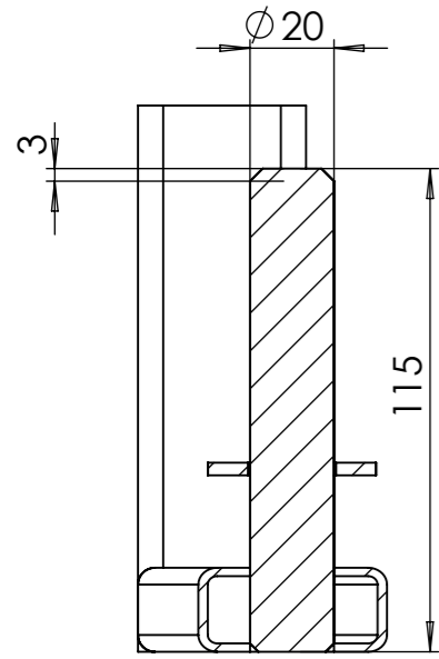
COUPE B-B ECHELLE 1 : 2
