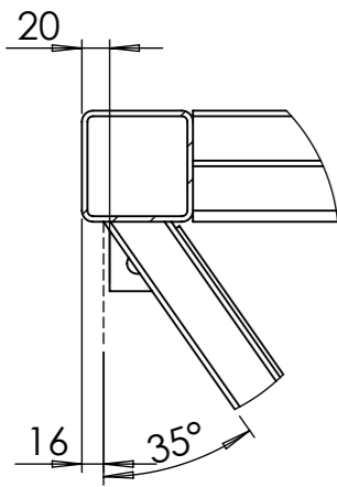
DÉTAIL E ECHELLE 1 : 6
