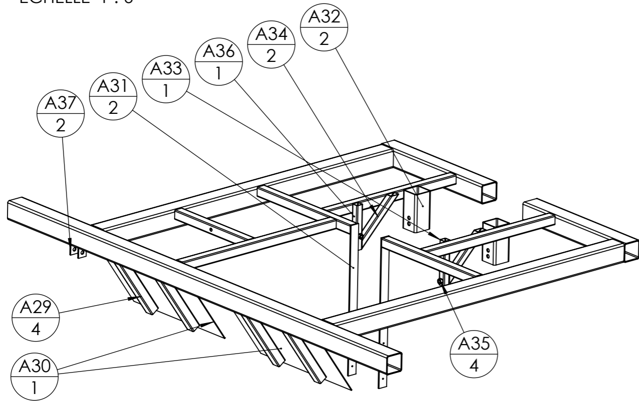
DÉTAIL E ECHELLE 1 : 6
