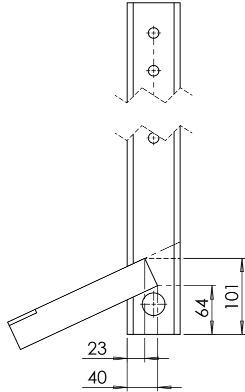
Version droite
