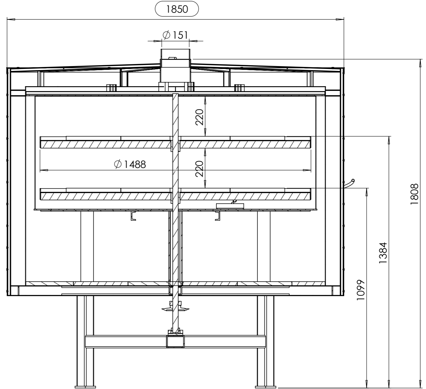
COUPE A-A
