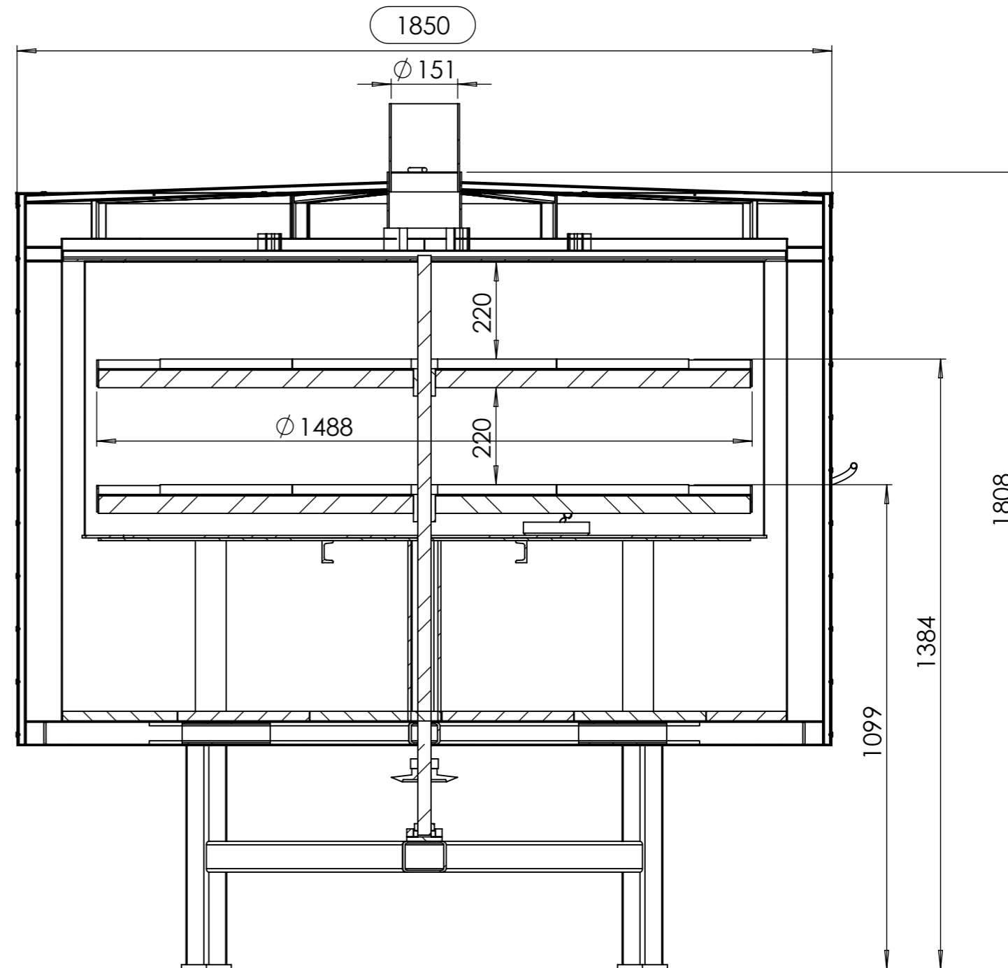
COUPE A-A
