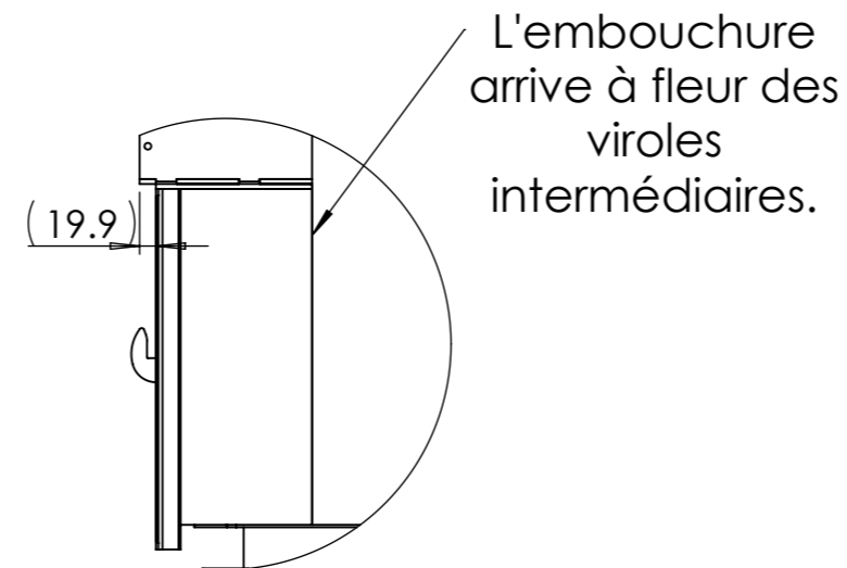
DÉTAIL ○ ECHELLE 1 : 10
