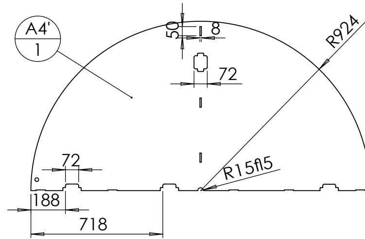
Epaisseur 3mm
