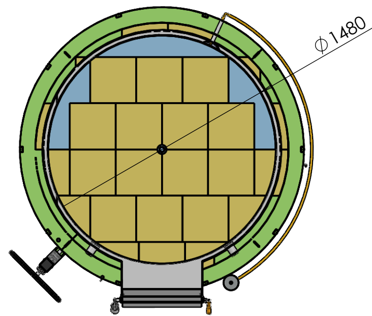
COUPE V-V ECHELLE 1 : 25
