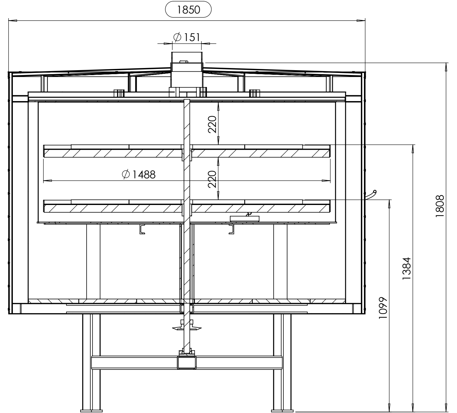
COUPE A-A
