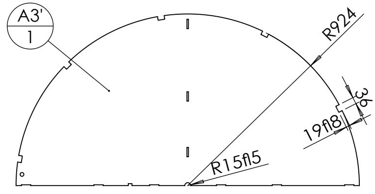
Epaisseur 3mm
