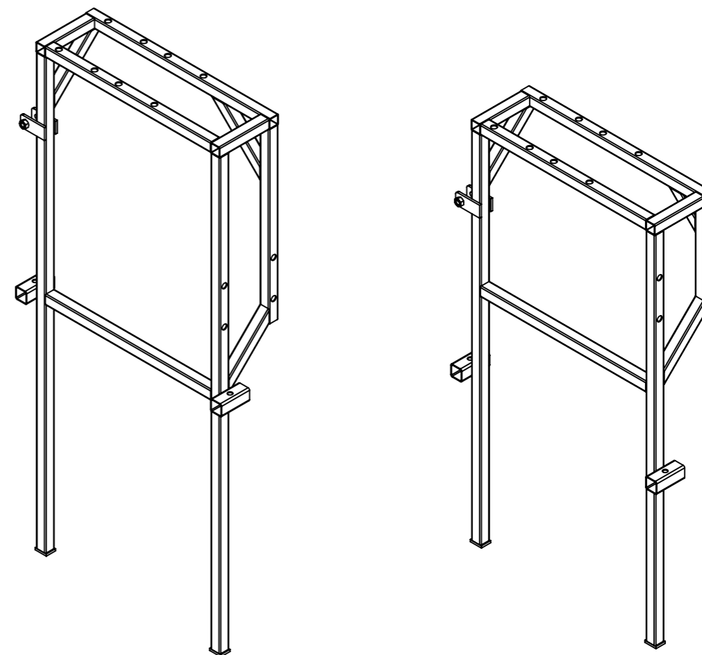
Aperçu des adaptations morphologiques de châssis
