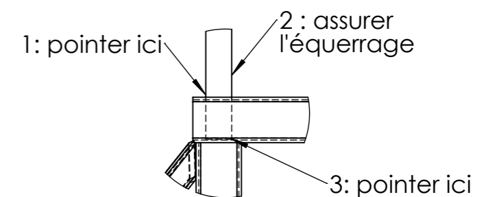
DÉTAIL B
