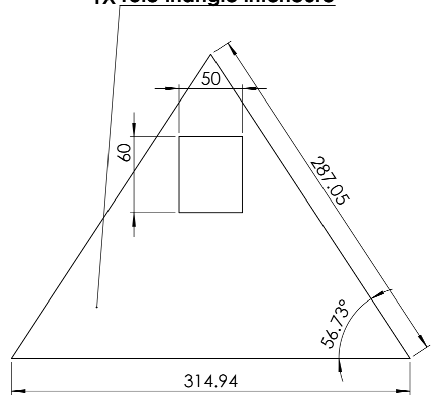
1X Tôle triangle intérieure
