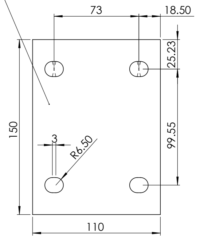
2X BA2 - Platine roue de jauge Herse
