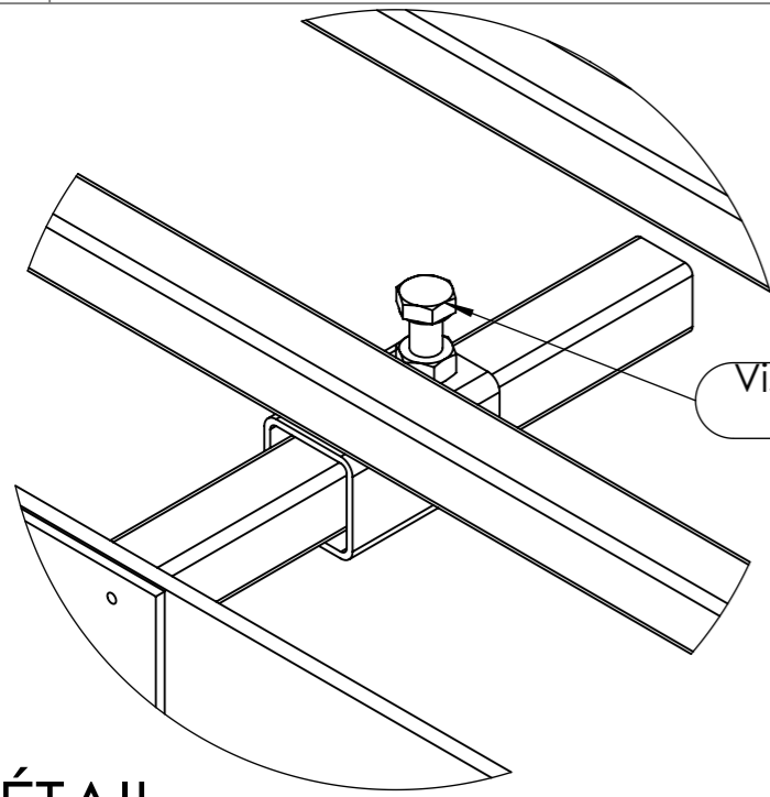
DÉTAIL M ECHELLE 1 : 2
