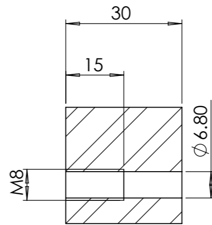
COUPE A-A ECHELLE 1 : 1
