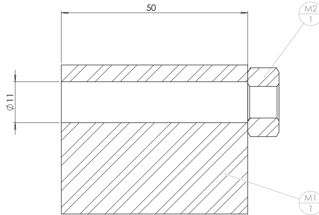
COUPE A-A EHELLE 2 : 1
