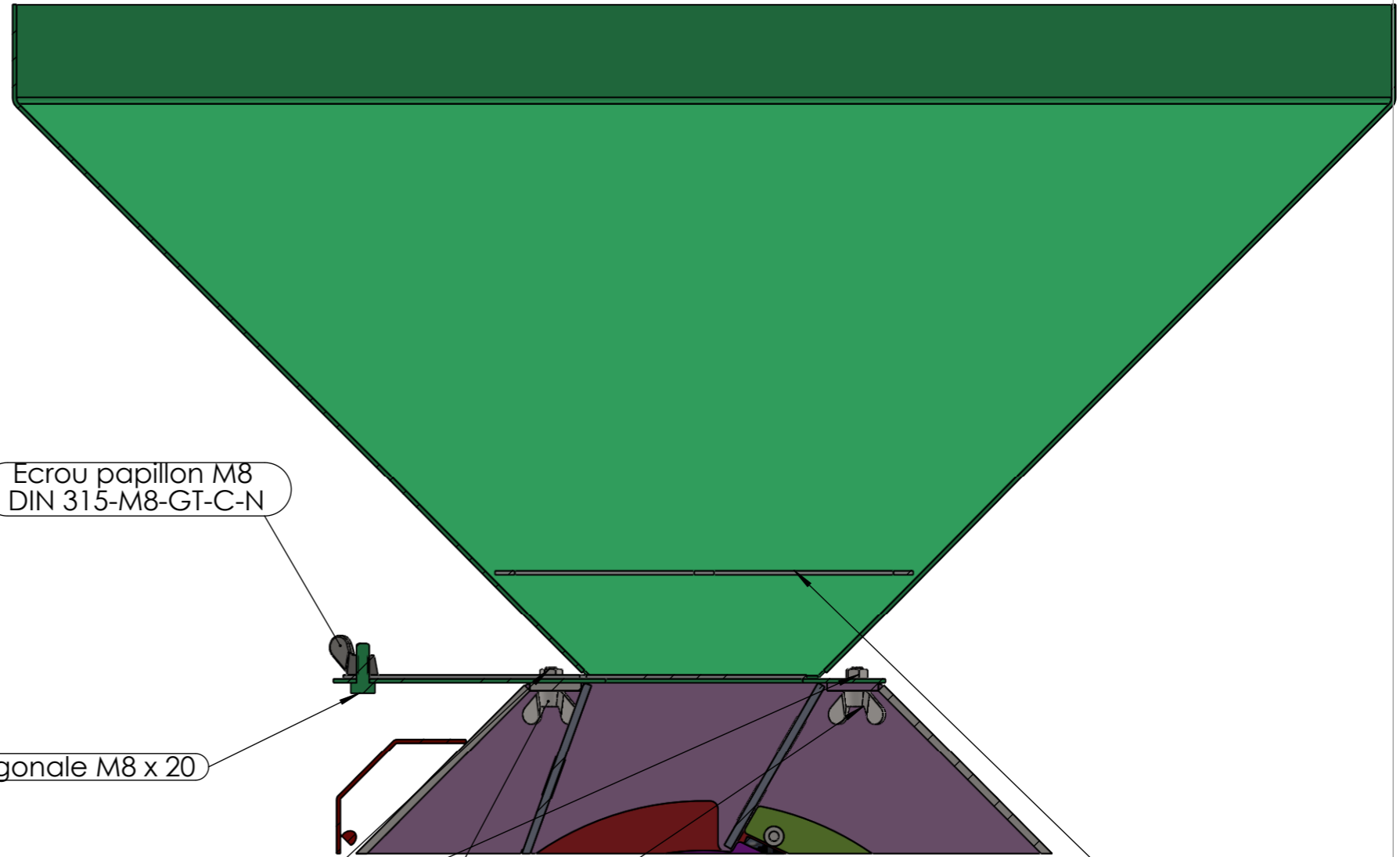
COUPE A-A ECHELLE 1 : 3
