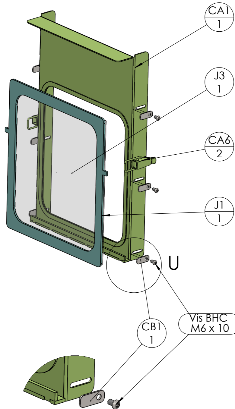
DÉTAIL U ECHELLE 2 : 5
