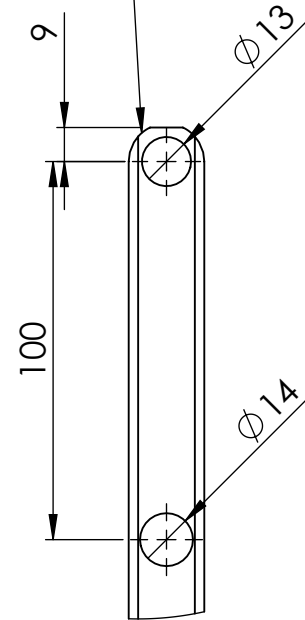
DÉTAIL Y ECHELLE 1 : 2
