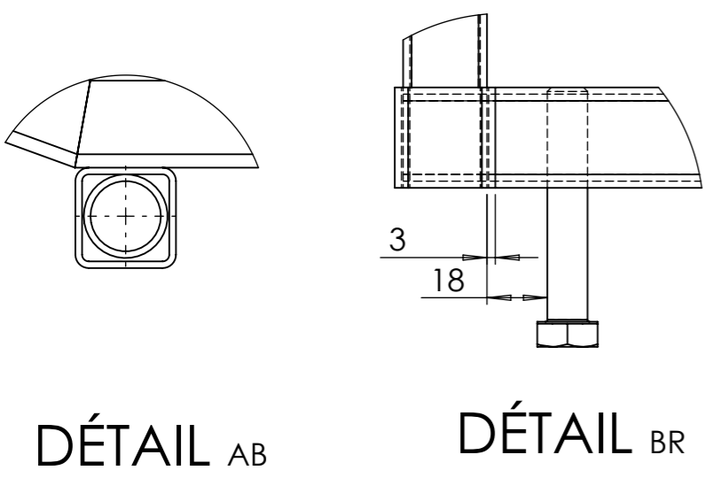
Support de béquille avant
