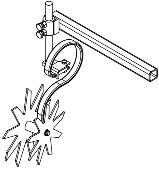
V - Roulémiette flanc de butte
