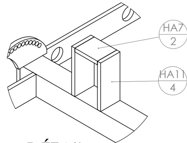
DÉTAIL A ECHELLE 1 : 5
