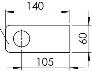
1X HA6 - plat flanc droit herse étrille
