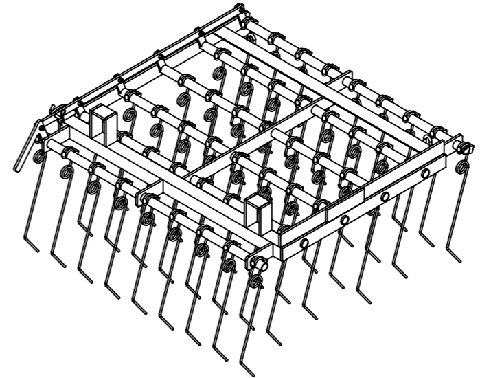
H - Cadre de herse
