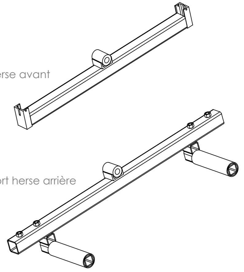
H - Cadre de herse
