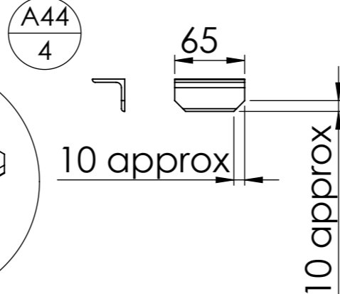
DÉTAIL SC ECHELLE 1 : 3
