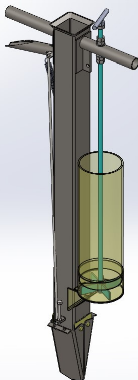
Canne à planter 60
