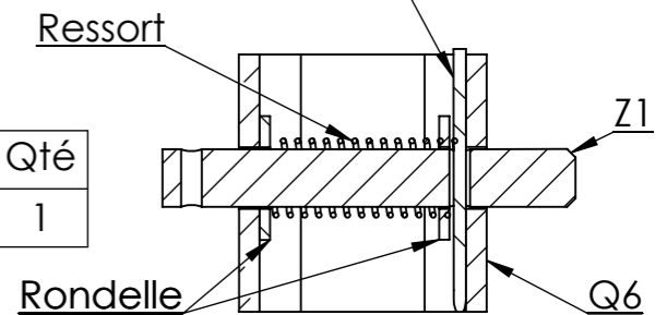
COUPE C-C ECHELLE 1 : 2
