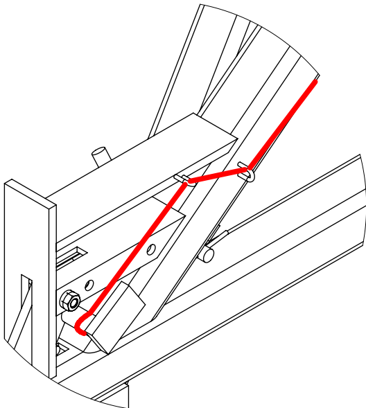
DÉTAIL A
