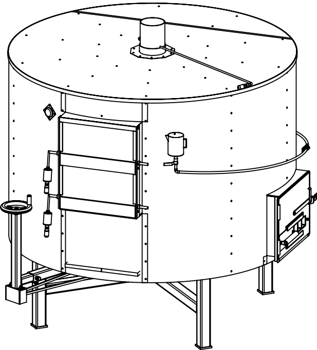
Version Foyer à 90° à droite
