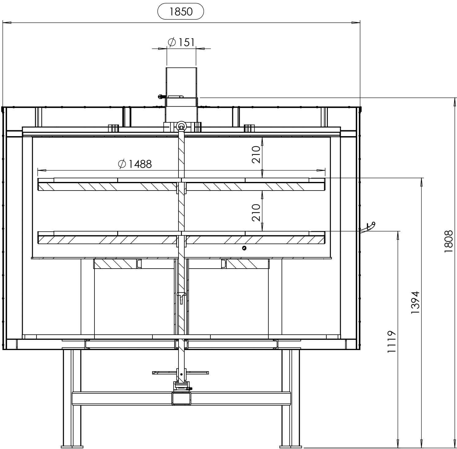
COUPE A-A
