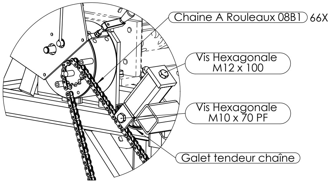
DÉTAIL B
