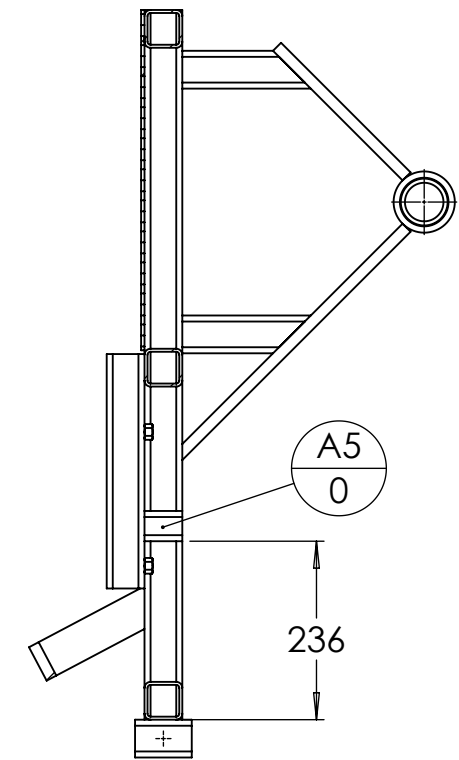
COUPE M-M ECHELLE 1 : 10
