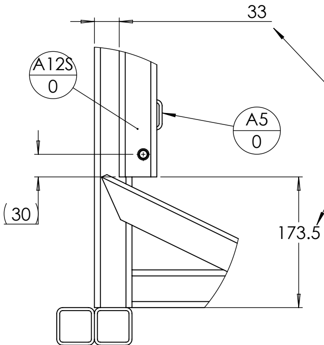
DÉTAIL P
