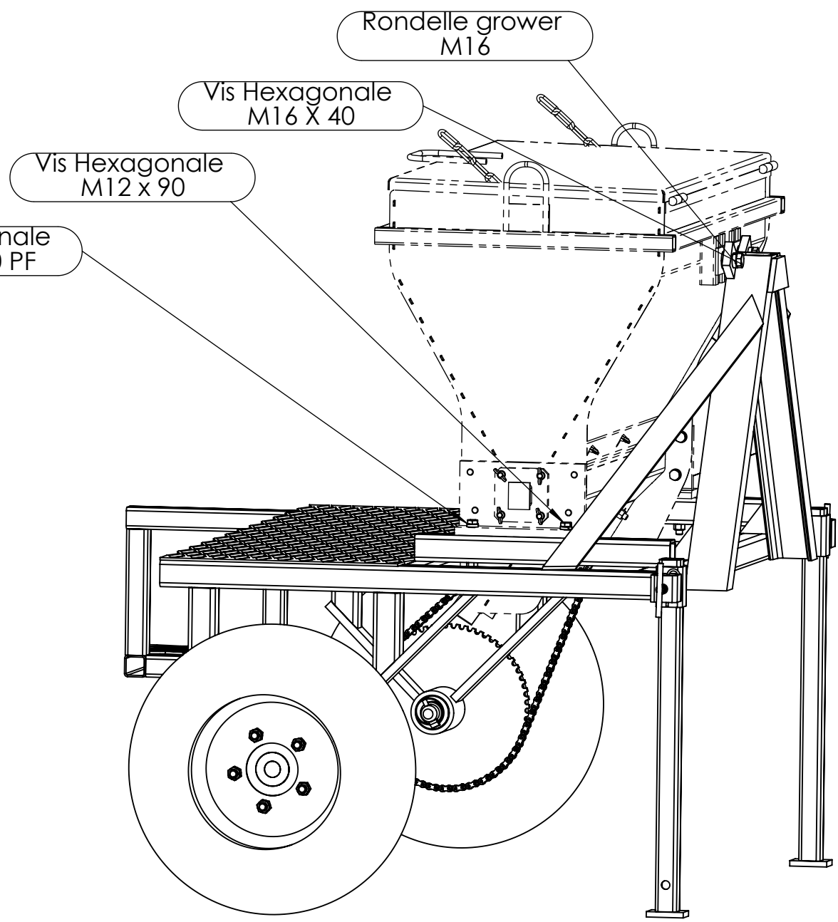
DÉTAIL Z
