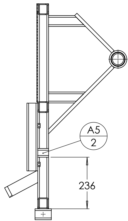
COUPE M-M ECHELLE 1 : 10
