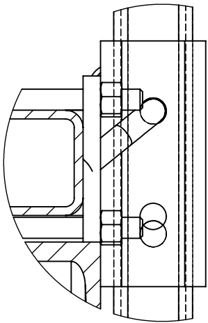
DÉTAIL B ECHELLE 1 : 3
