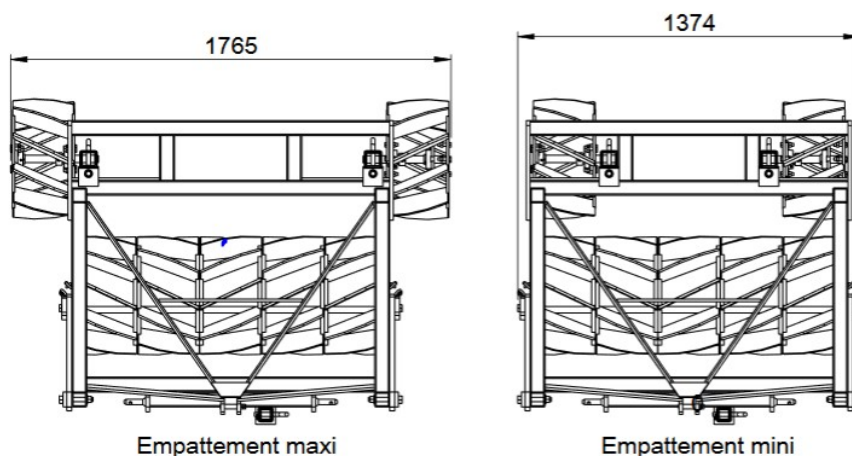
Illustration de la variation de la largeur par les roues de jauge, 5 roues de travail "250" et 2 roues de jauges "250".
