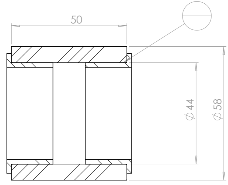
COUPE E-E ECHELLE 1 : 1
