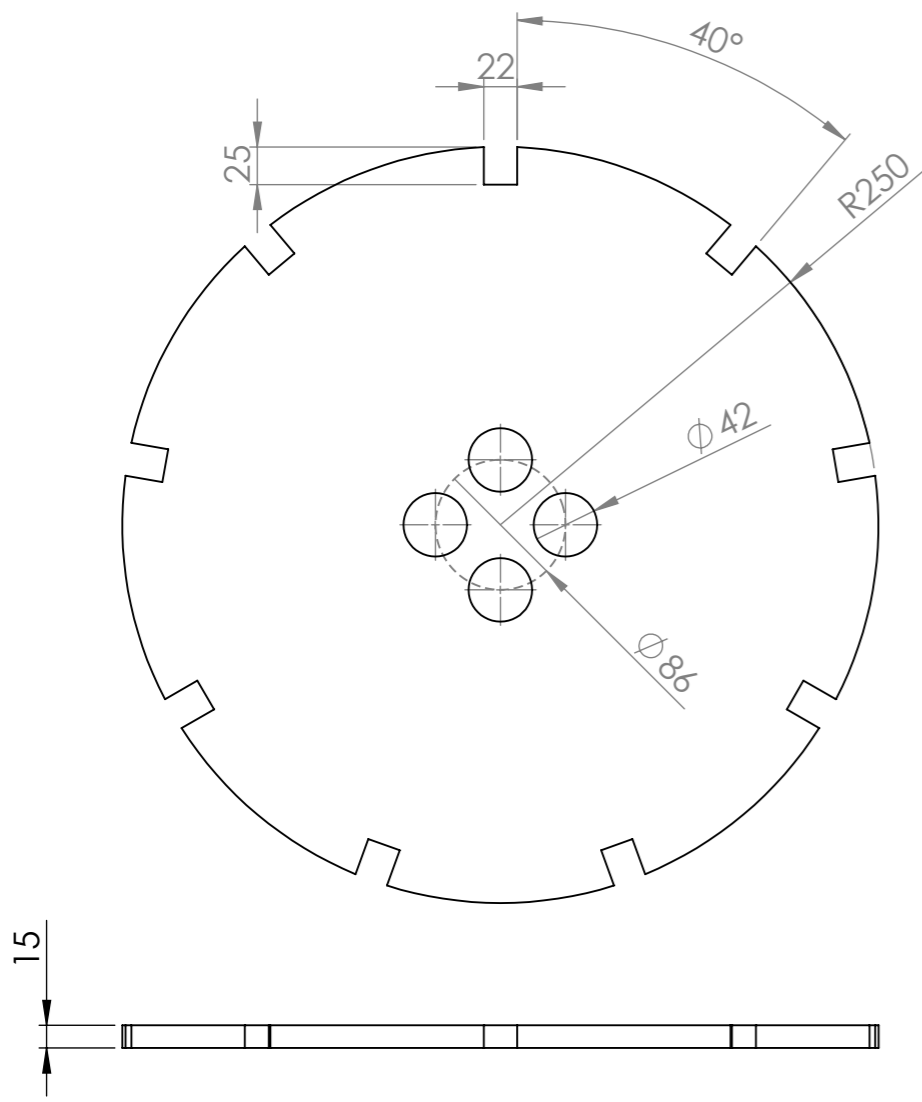
Disque central
