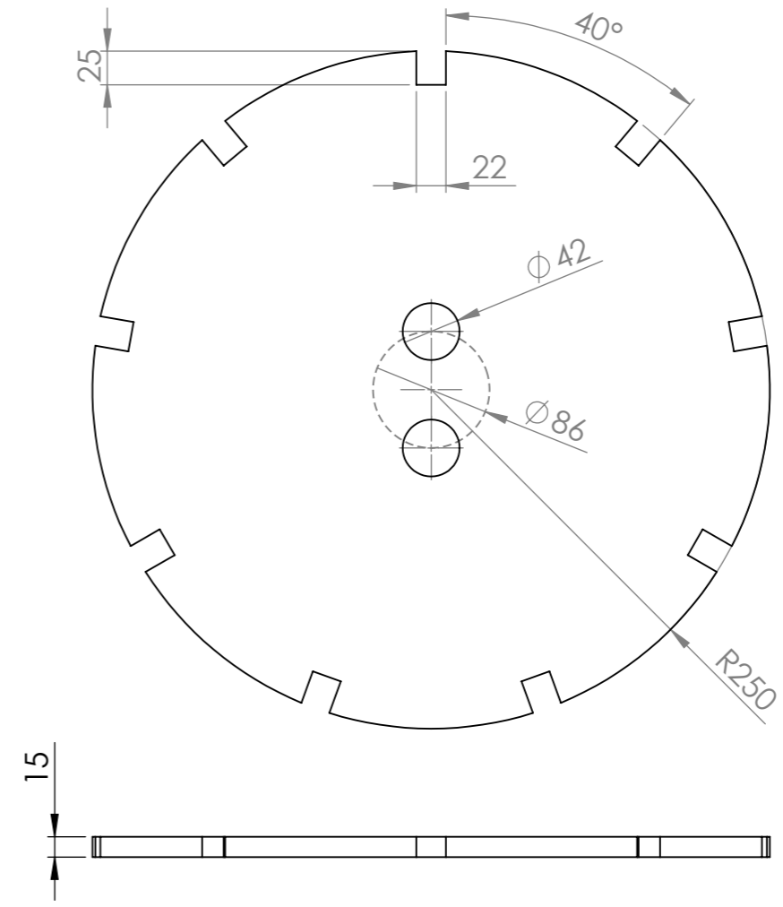
Disque externe
