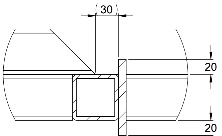
DÉTAIL B
