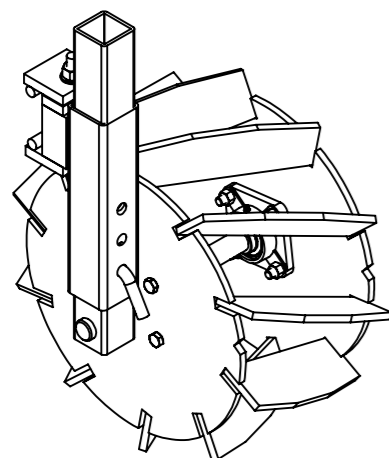
Ensemble Jauge 250
