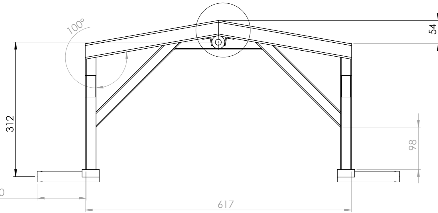
Détail S
