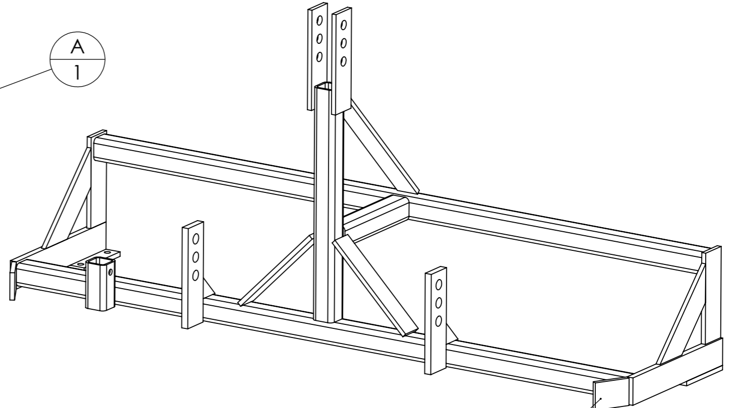
A - Bati Rouleau
