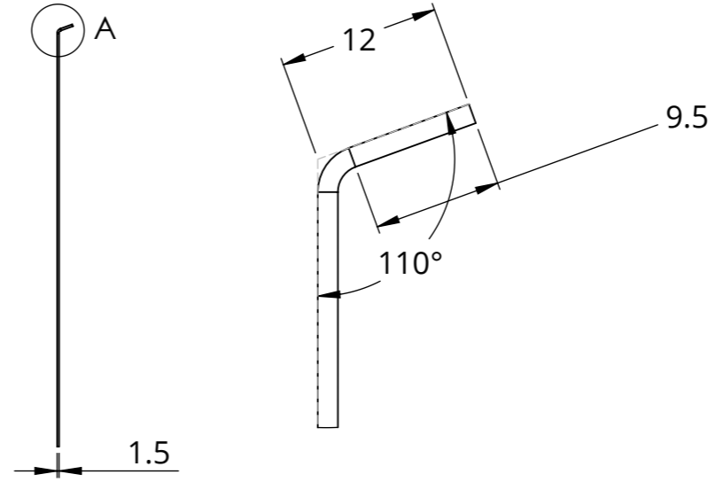
DÉTAIL A
