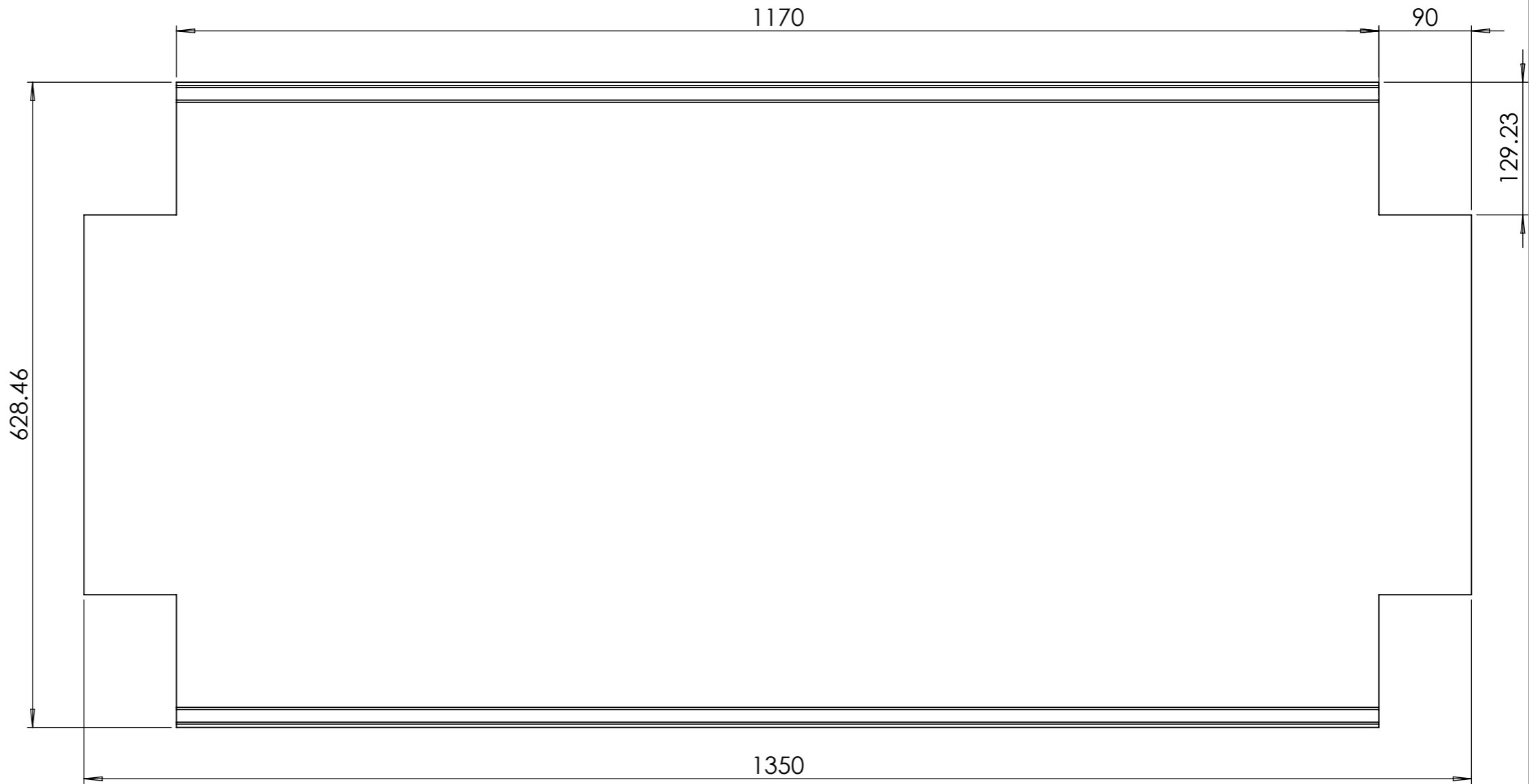
DÉTAIL C ECHELLE 1 : 1
