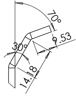
DÉTAIL C ECHELLE 1 : 1
