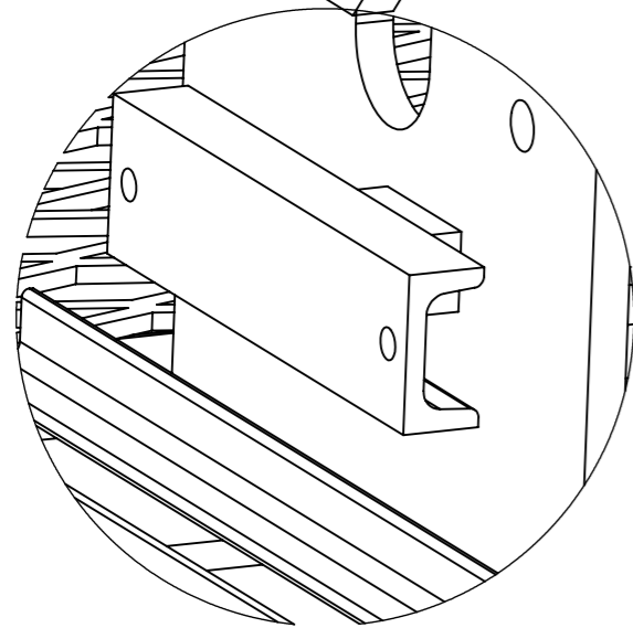
DÉTAIL G ECHELLE 1 : 2
