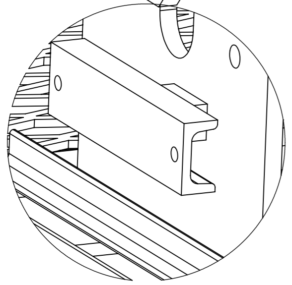
DÉTAIL G ECHELLE 1 : 2
