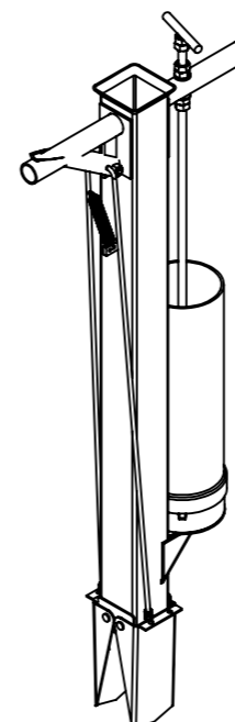
Canne à planter Tube central de 60 Levier unique
