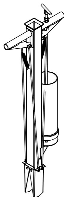
Canne à planter Tube central de 50 Double levier
