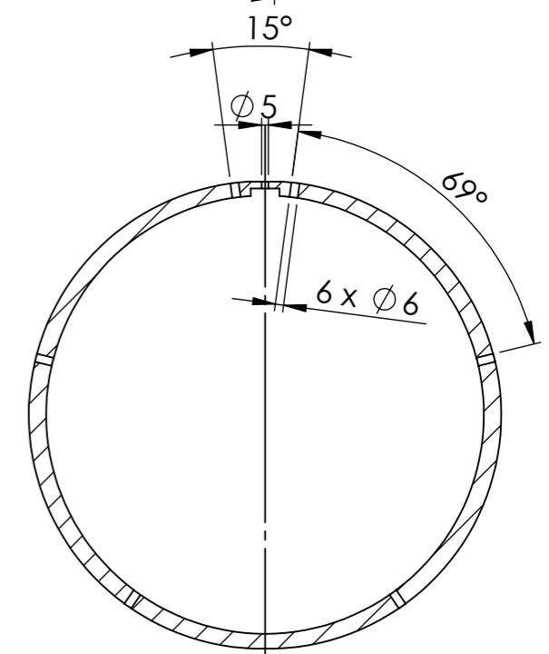
Pièce réalisée en découpe laser (fichier disponible sur notre site)
