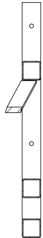
COUPE C-C ECHELLE 1 : 10
