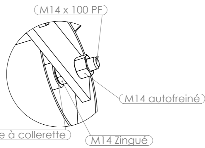
DÉTAIL A ECHELLE 2 : 5 Fixation de la roue
