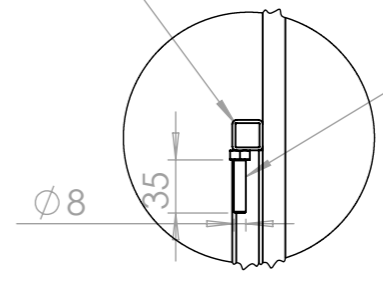
DÉTAIL E ECHELLE 1 : 5
