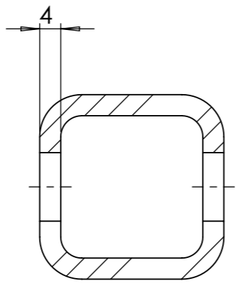
COUPE A-A
