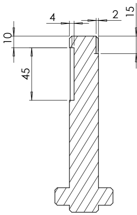
COUPE B-B
