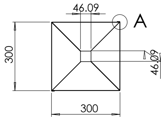
DÉTAIL A ECHELLE 1 : 1
