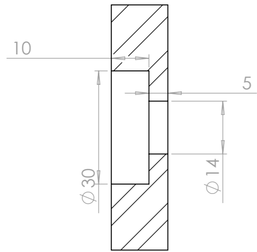
COUPE A-A
