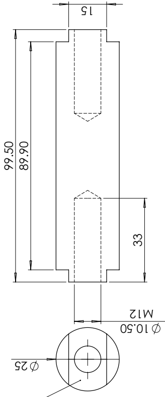
Axe double pour étoiles \phi 25 L99.5
