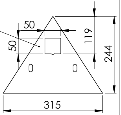
A3 1 Acier S235 Epaisseur 8mm
