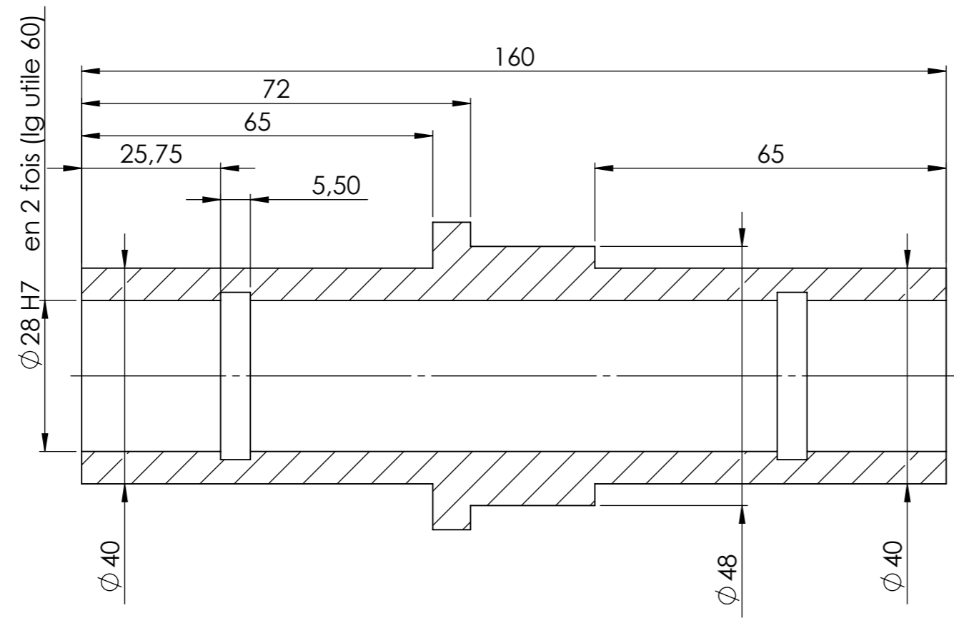
COUPE A-A
