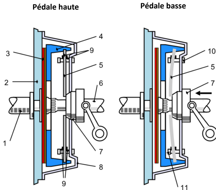
1-Arbre moteur 2-Volant moteur 3-Disque d'embrayage 4-Plateau mobile 5-Diaphragme 6-Arbre de sortie 7-Butée d'embrayage 8-Couvercle 9-Jonc 10-Colonnes de fixation 11-Collet d'arrêt
