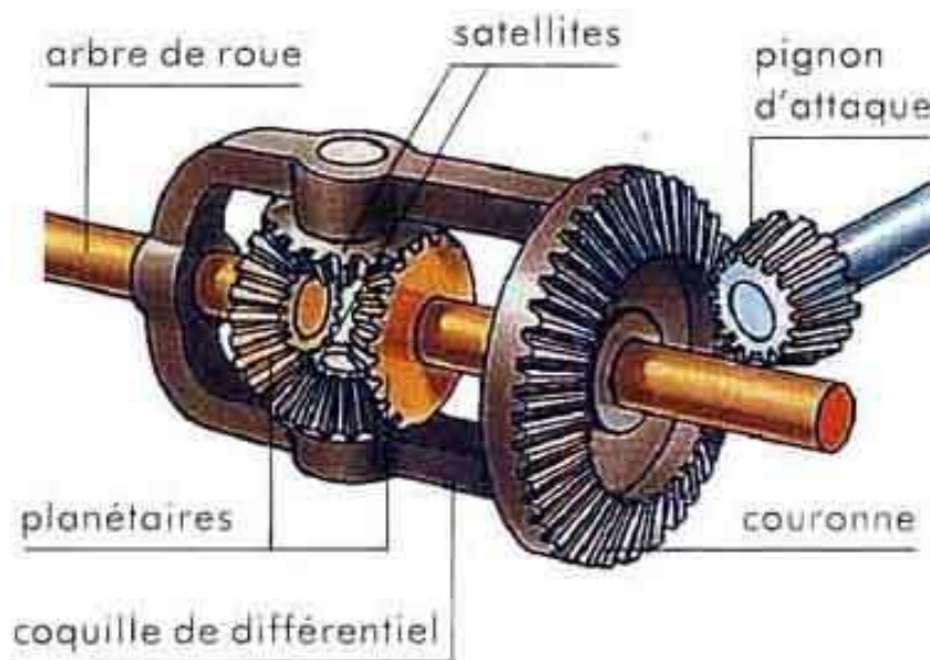
Figure 7: Bloc différentiel
