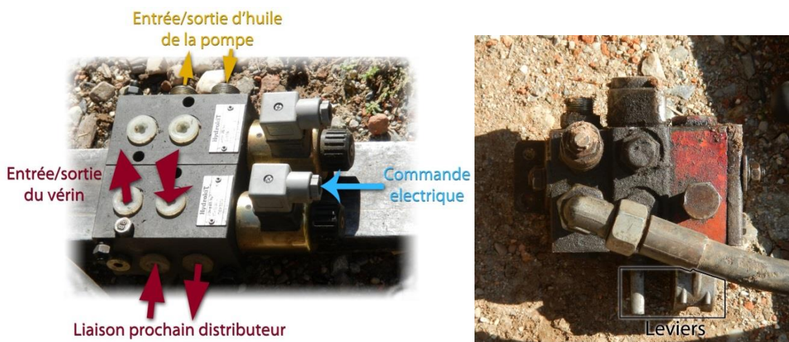
Figure 10: Distributeurs électriques (à gauche) et mécaniques (à droite)
