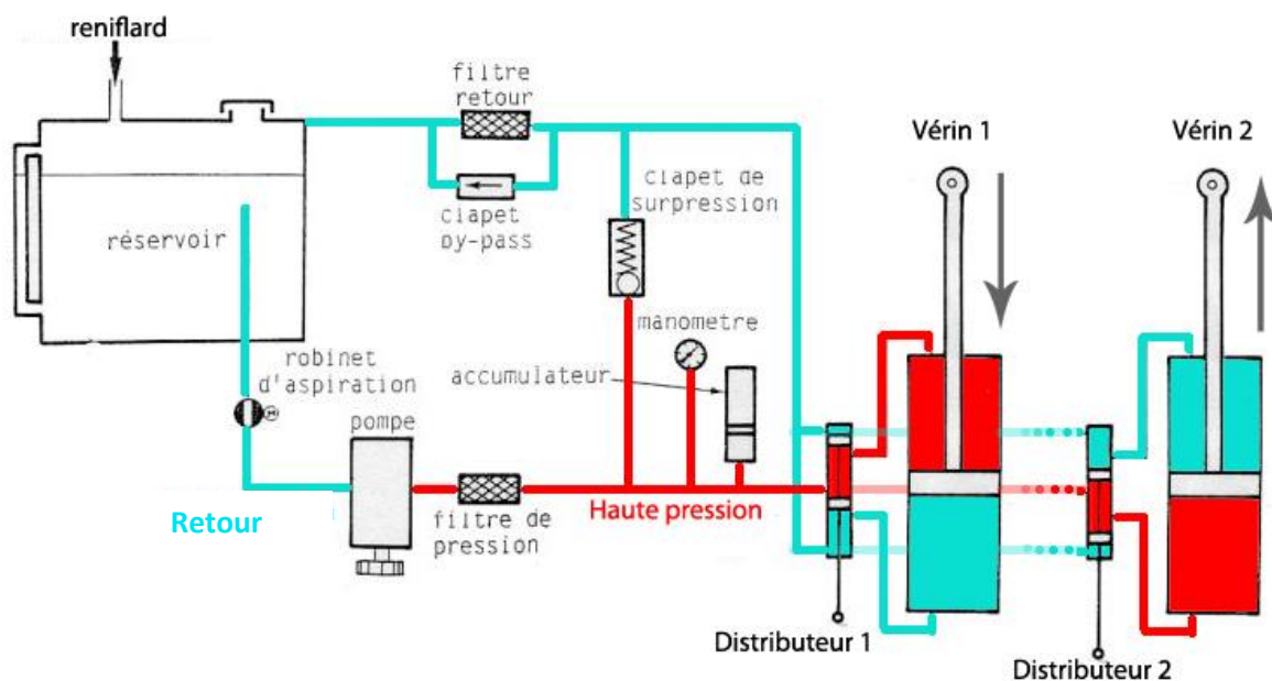
Figure 9: Schéma du circuit hydraulique de tracteur
