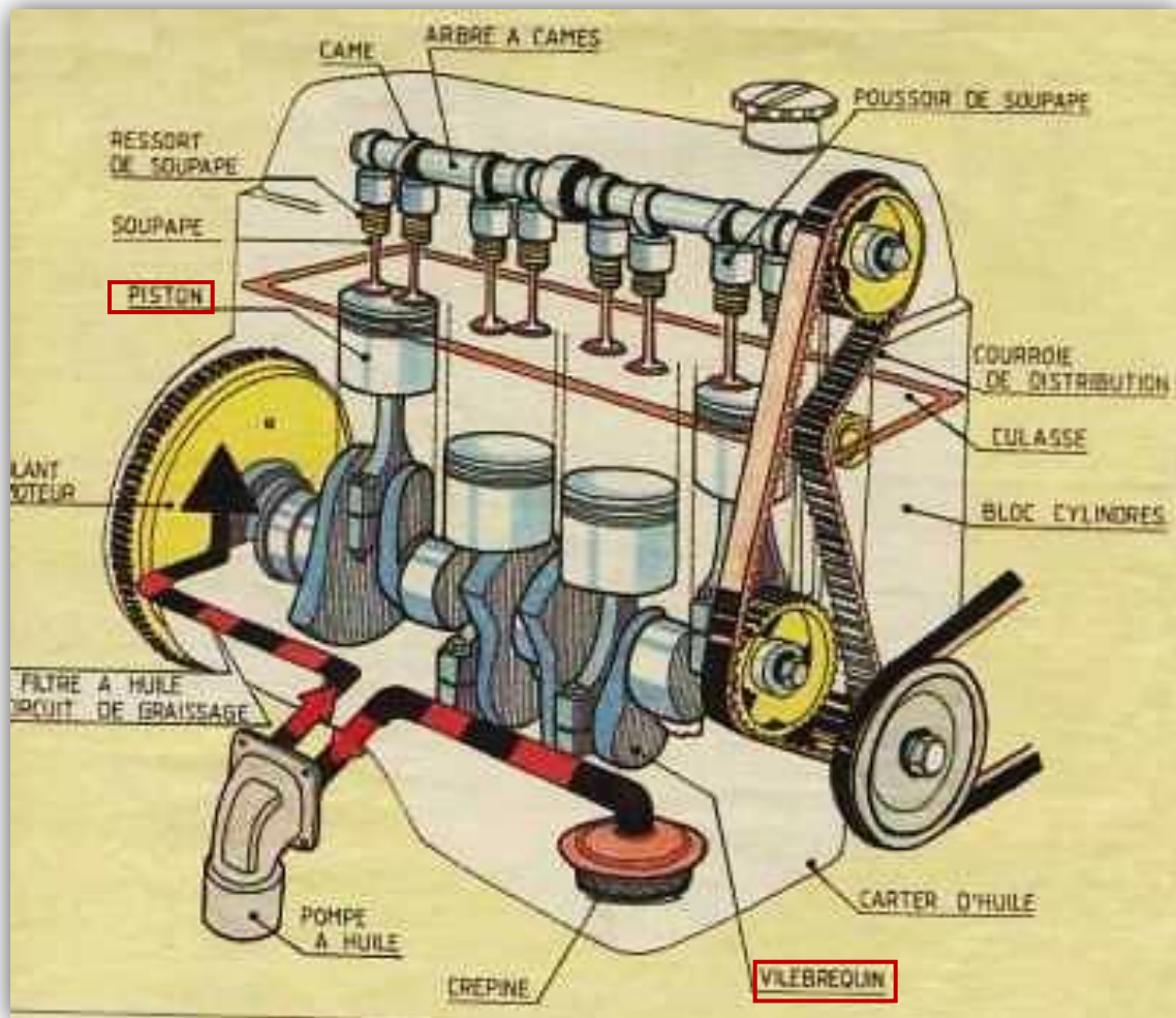
Figure 1: Schéma d'un moteur à 4 temps
