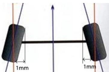
Figure 4: Réglage du parallélisme (4 RM)
