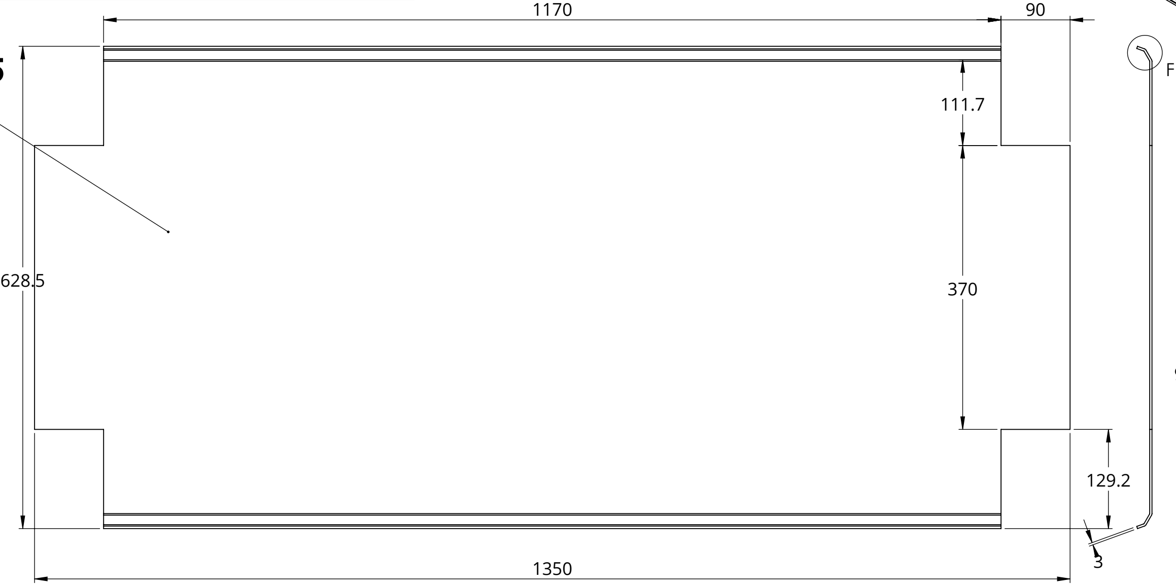
Déplié indicatif (cote pliées fonctionnelles)
