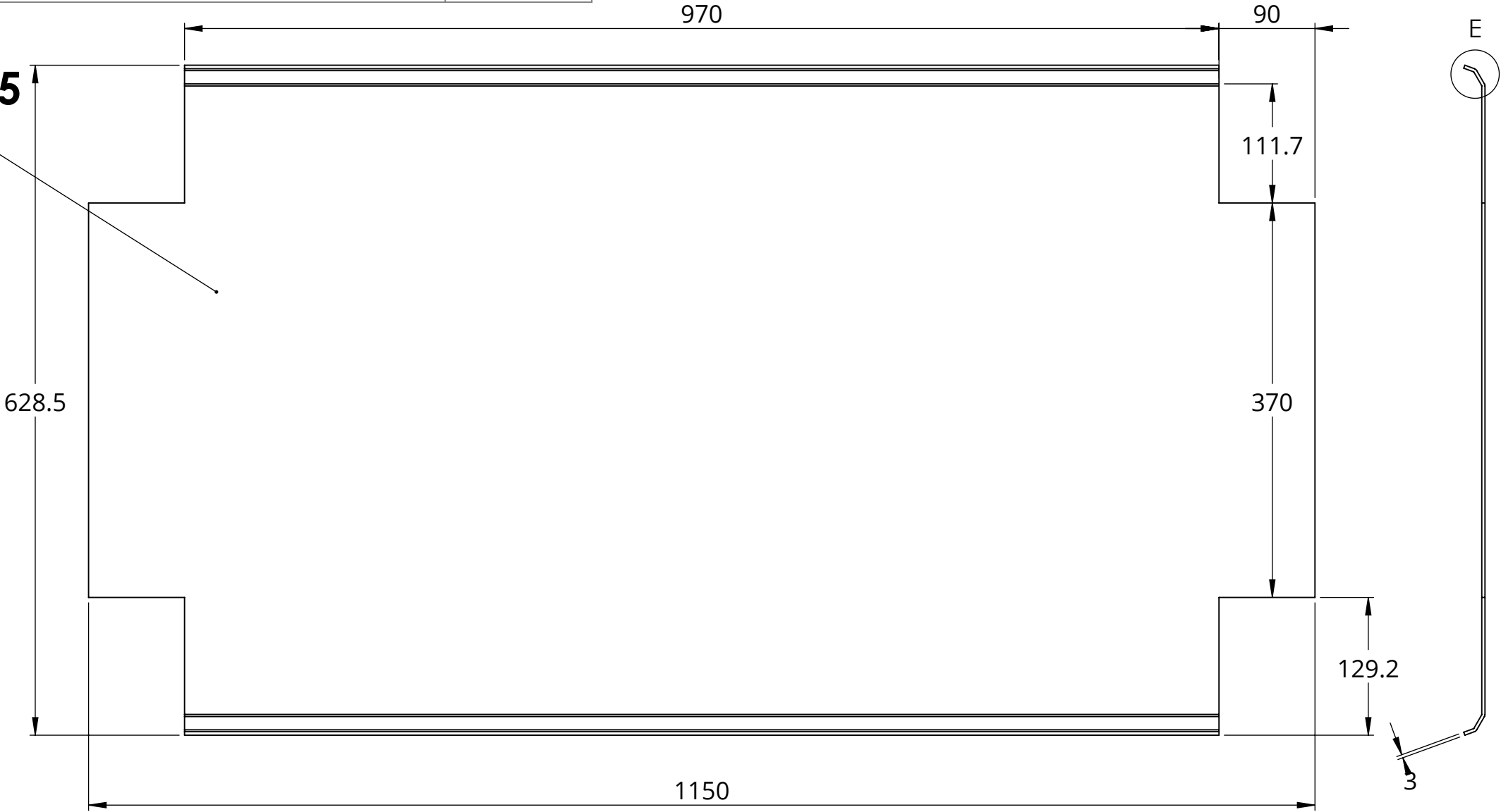
Déplié indicatif (cote pliées fonctionnelles)
