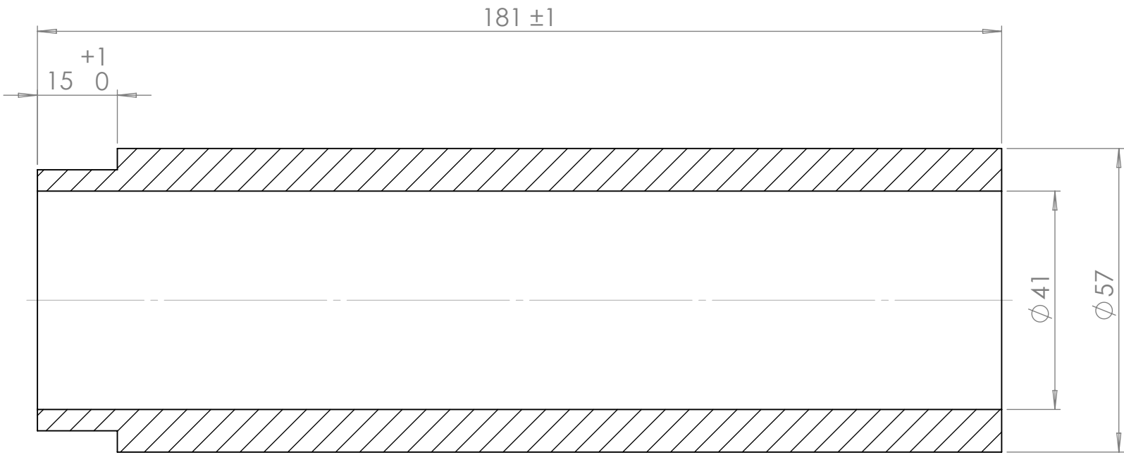
COUPE U-U ECHELLE 1 : 1
